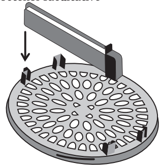
Installation de la bande à l'octenol facultative
